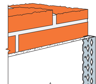
PEB Plasterboard Edge Bead
