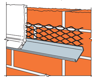
ERS Render Stop Bead
